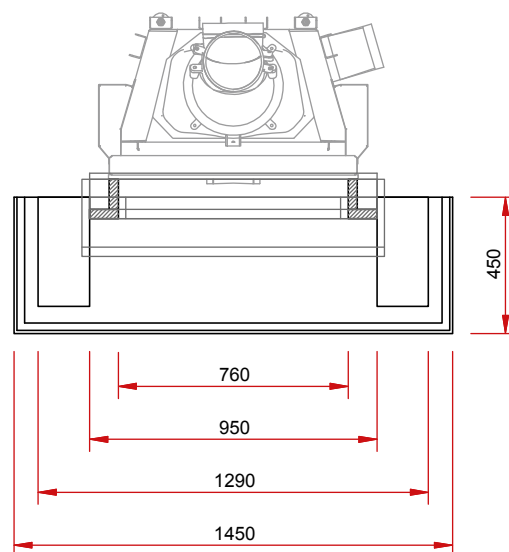
Изображение сверху М 1:25
