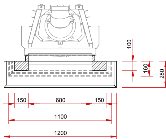
Изображение сверху М 1:25
